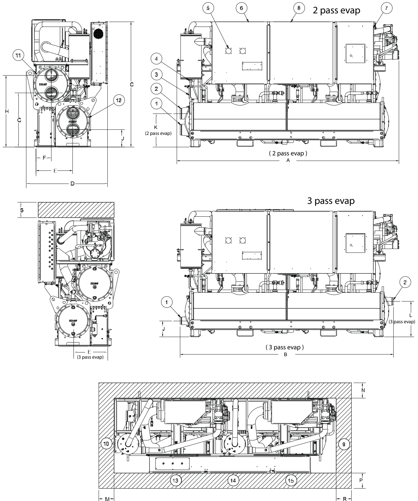
Figure 7. RTWD - 50 Hz dimensions - 130-250 ton HE, 160-200 ton PE
