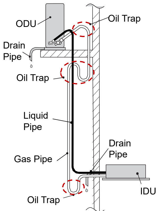
Unidad exterior instalada por arriba de la unidad interior
