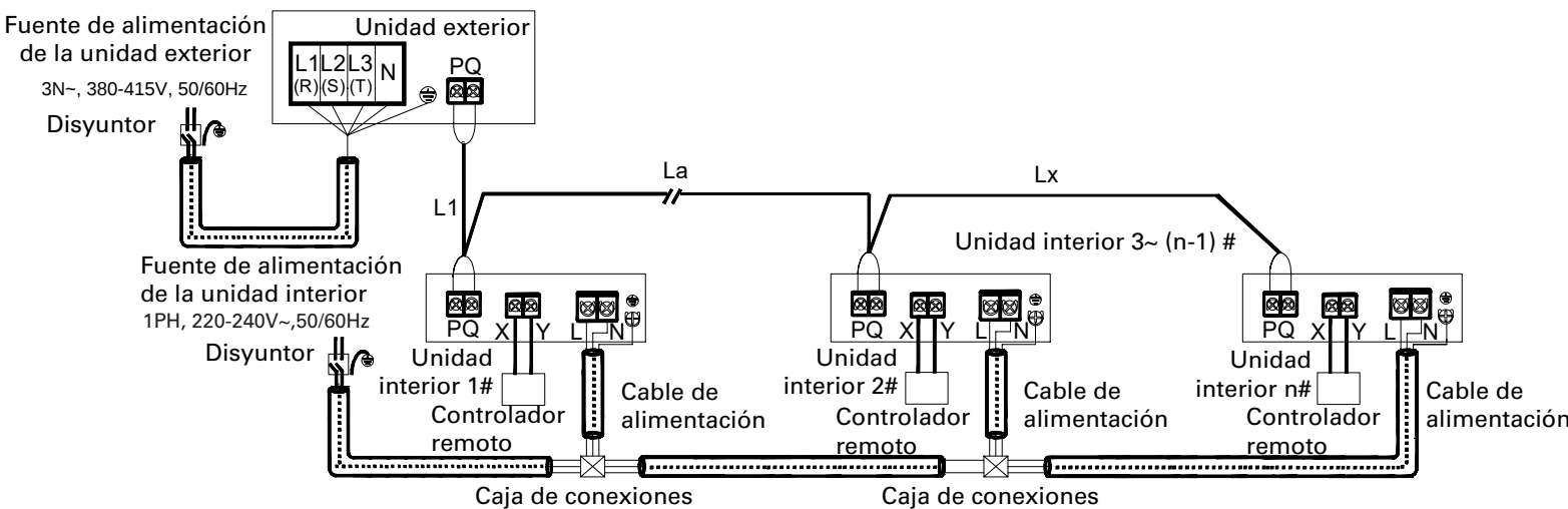
Figura del cableado de alimentación
