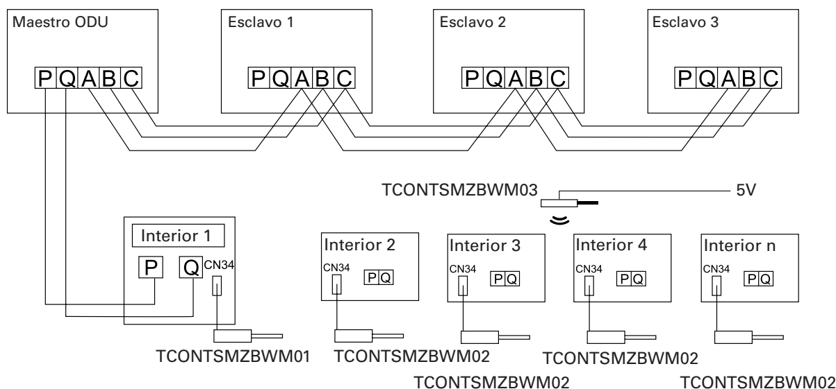
Figura de cableado de comunicación (inalámbrica)
