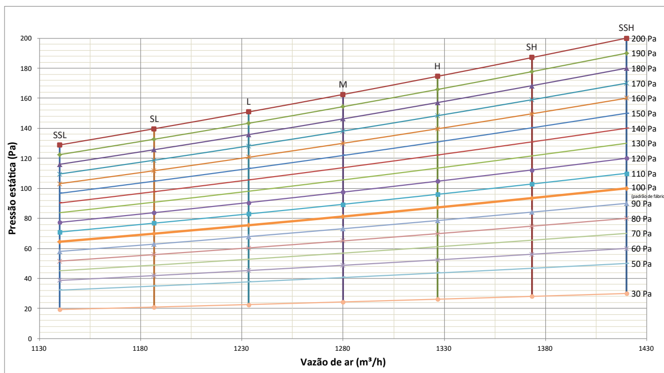
Figura 12: Desempenho do ventilador do 4TVA0030EF000AA
