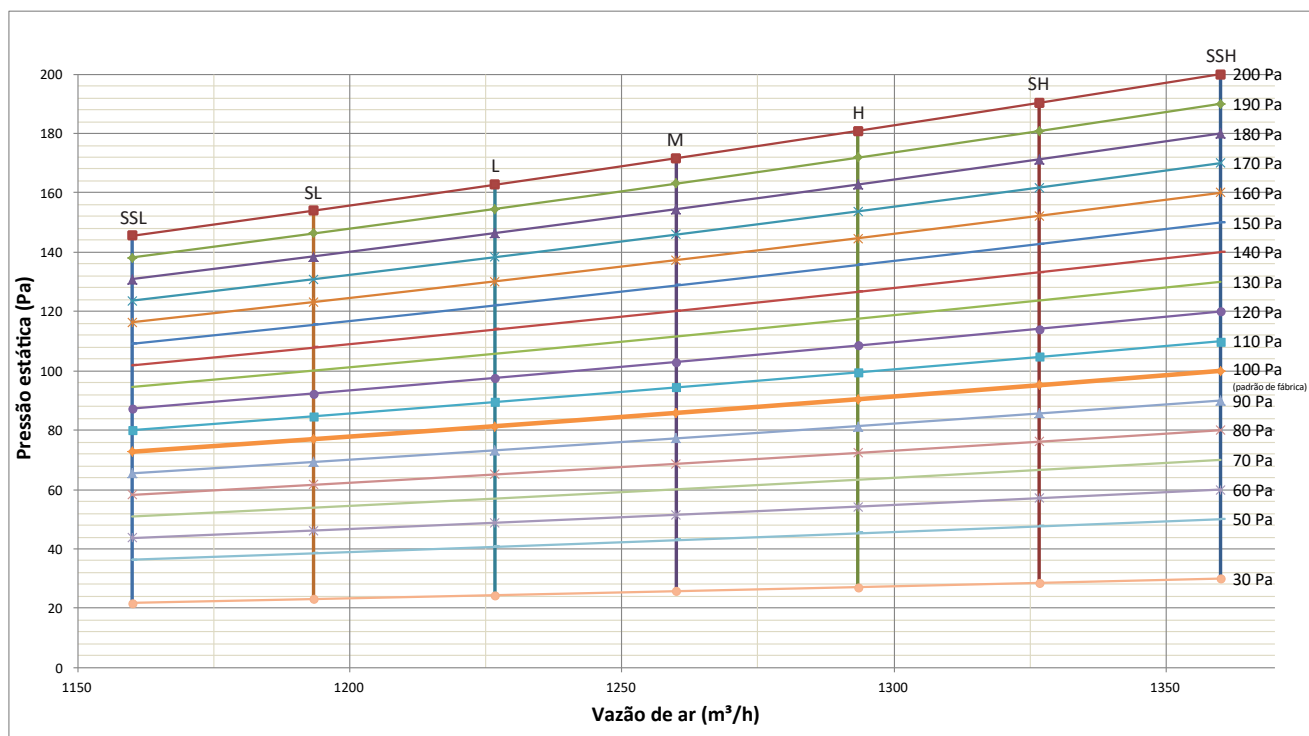
Figura 11: Desempenho do ventilador do 4TVA0024(27)EF000AA
