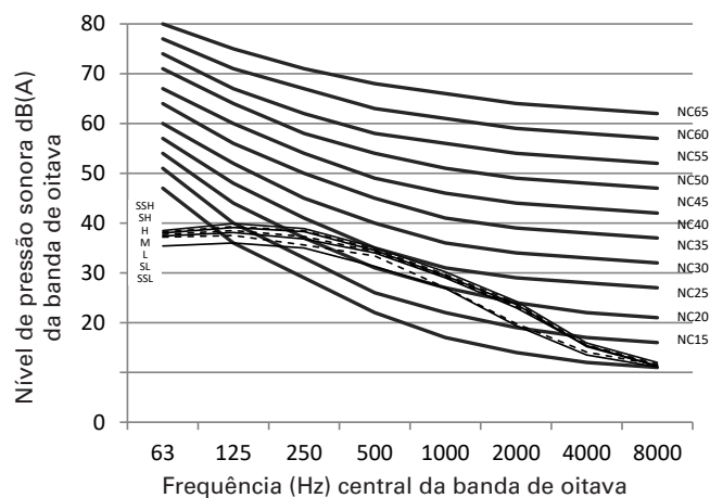
Figura 25: Níveis da banda de oitava do 4TVA0192EF000AA
