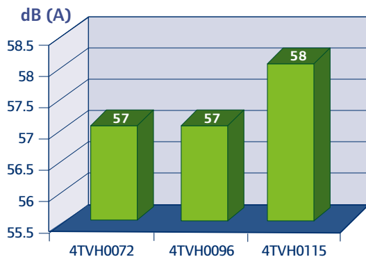
Presión de sonido a 3.28 pies exteriores
