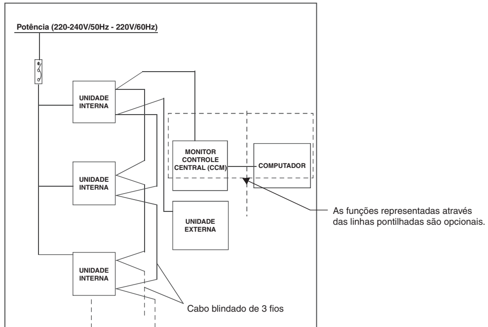
Figura 19. Esquema de Cabeamento
