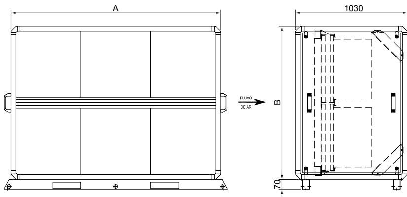
Fig. XVII-13 - Cotas Módulo Filtro de Retorno WD/WL - F8 Bolsa + 1" ou apenas F8 Bolsa (10 a 40) Siroco e Limit Load
