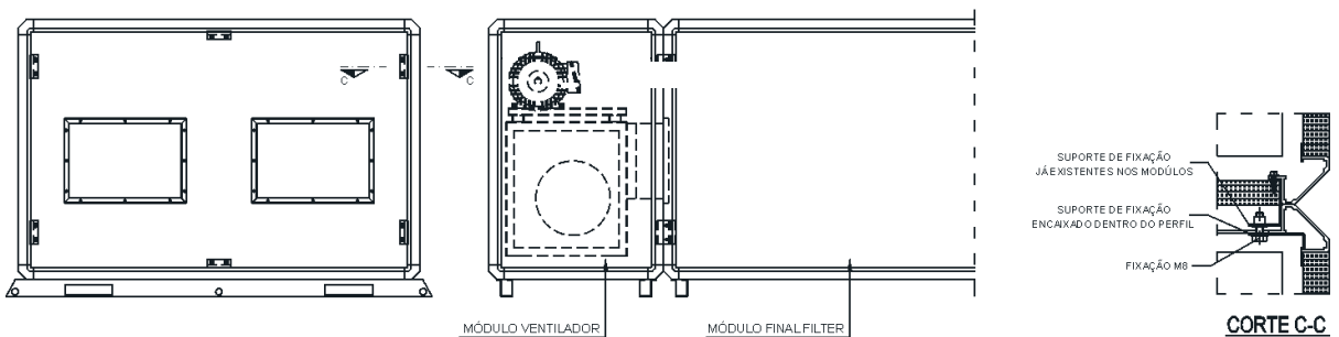
Fig. XVII-22 - Montagem Horizontal com Final Filter
