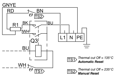
DETAGLIO COLLEGAMENTO ELETTRICO ELECTRIC HEATER WIRING DETAIL DÉTAILS RACCORDEMENT ÉLECTRIQUE
