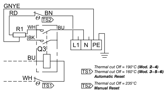
DETAIL DER ELEKTRISCHEN VERBINDUNG DÉTAILS CONEXIÓN ELÉCTRICA ELEKTRISCHE AANSLUITING DETAIL
