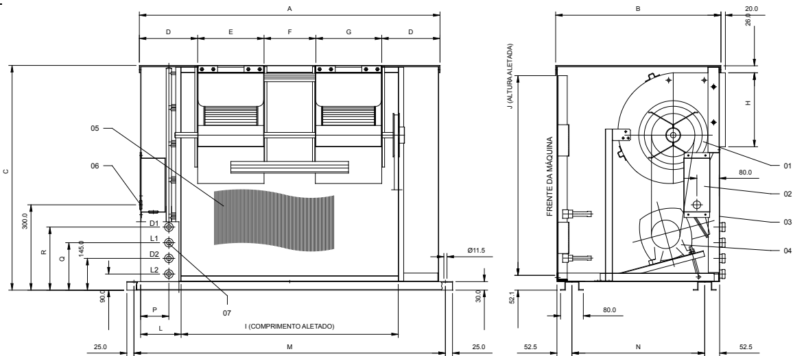
Fig. IX-11 - Dimensiones CRCB 050 a 150.
