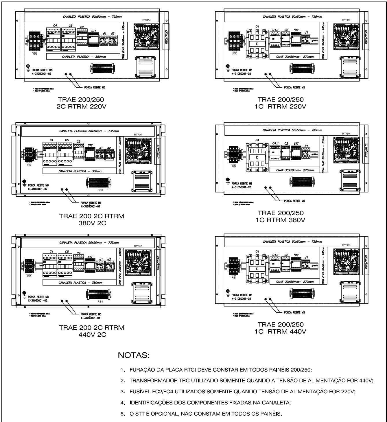
Fig. VII-19 - Lay Out de Tableros Eléctricos - TRAE (RTRM)
