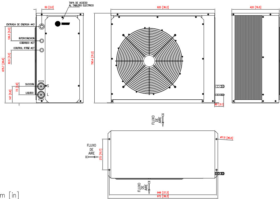
Fig. IX-02 - Dimensional Unidades Condensadoras TRAE 075
