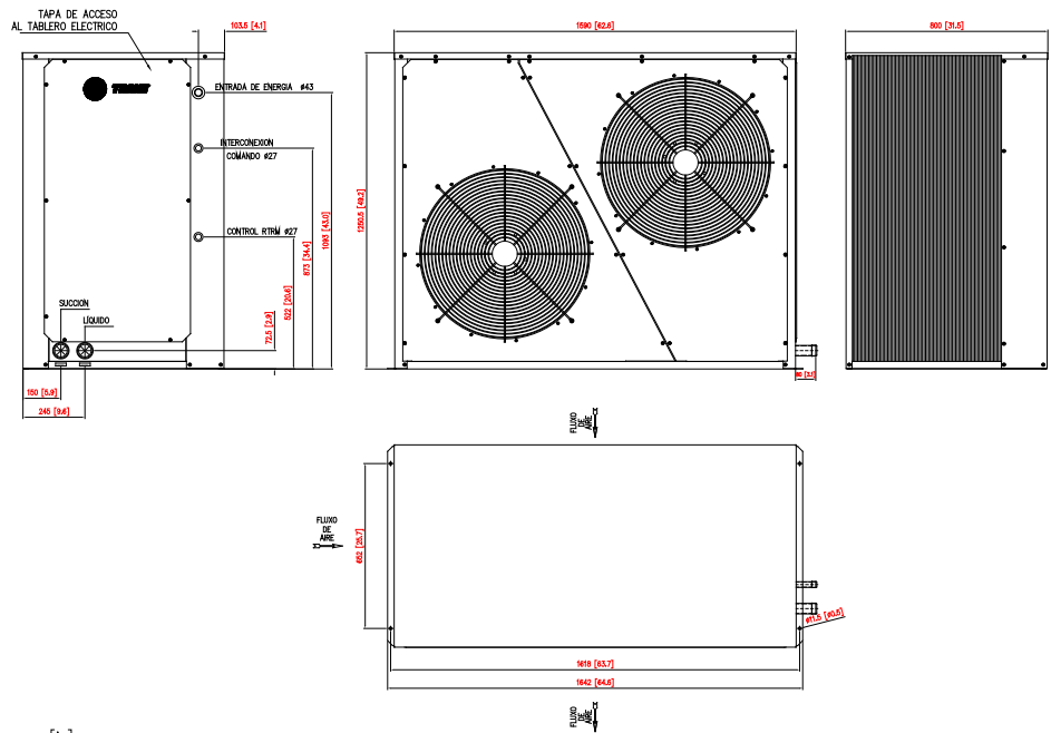
Fig. IX-05 - Dimensional Unidades Condensadoras TRAE 150 - 1 Circuito
