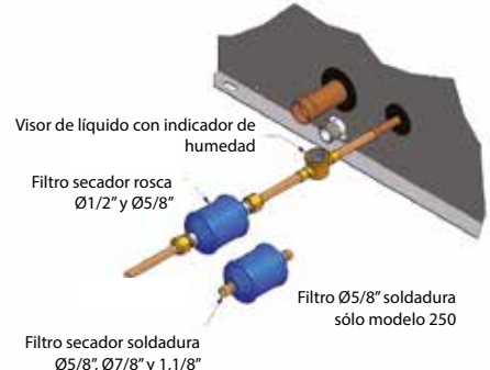
Esquema de montaje Filtro secador y visor de líquido
