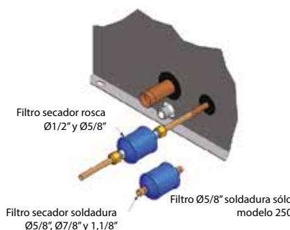
Esquema de montaje Filtro secador
