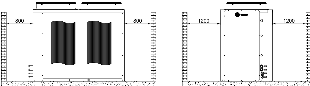
Fig. X-02 - Espacios sugeridos TRAE 200 a 250 - Descarga Vertical
