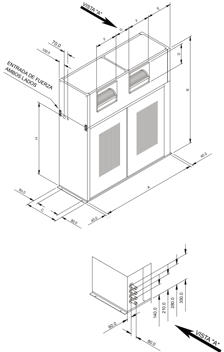
Fig. IX-13 - Datos Dimensionales TRCE/CRCE
