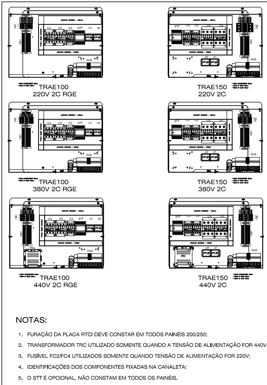
Fig. VII-20 - Lay Out de Tableros Eléctricos - TRAE (RGE)
