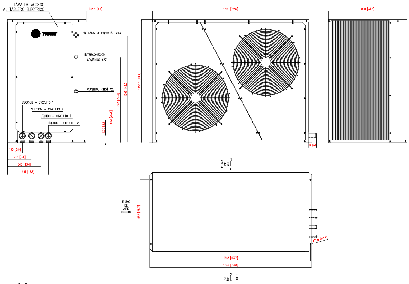
Fig. IX-06 - Dimensional Unidades Condensadoras TRAE 150 - 2 Circuitos
