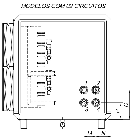
Fig. XVIII-11 - Circuitos de Refrigeração do Módulo Serpentina 10 a 50
