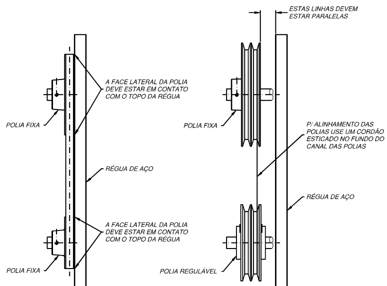
Fig. XVI-03 - Alinhamento das correias
