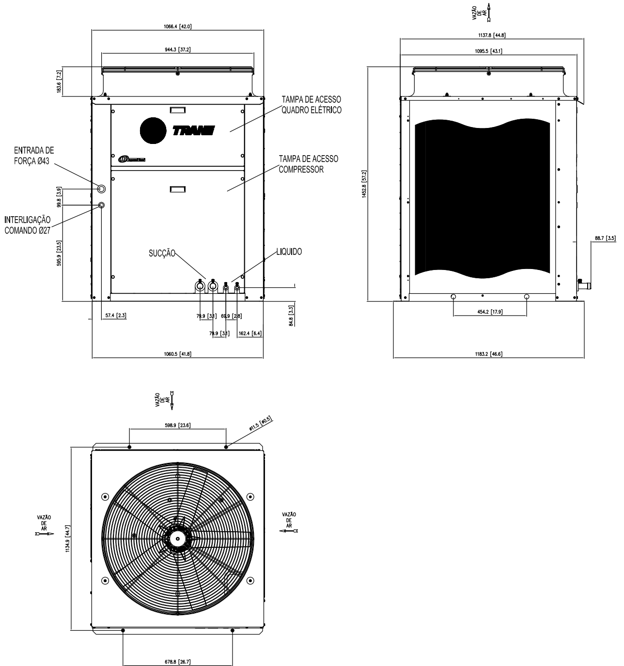
Fig. XVIII-36 - Dimensional Unidades Condensadoras TRAE 250 - 2 circuitos
