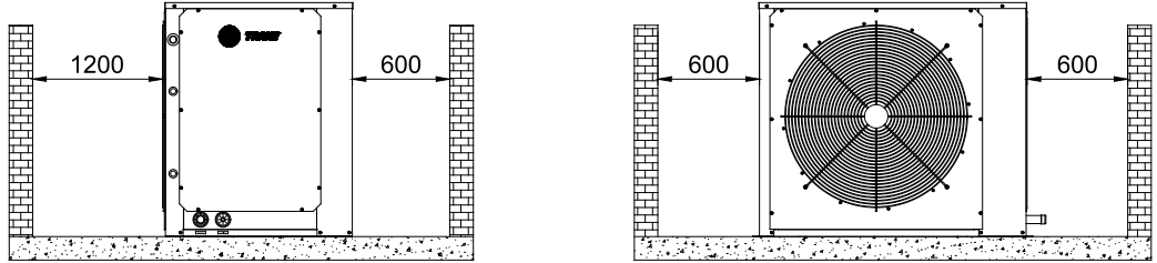
Fig. XVIII 39 - Espaços para Manutenção e Circulação de Ar - TRAE
