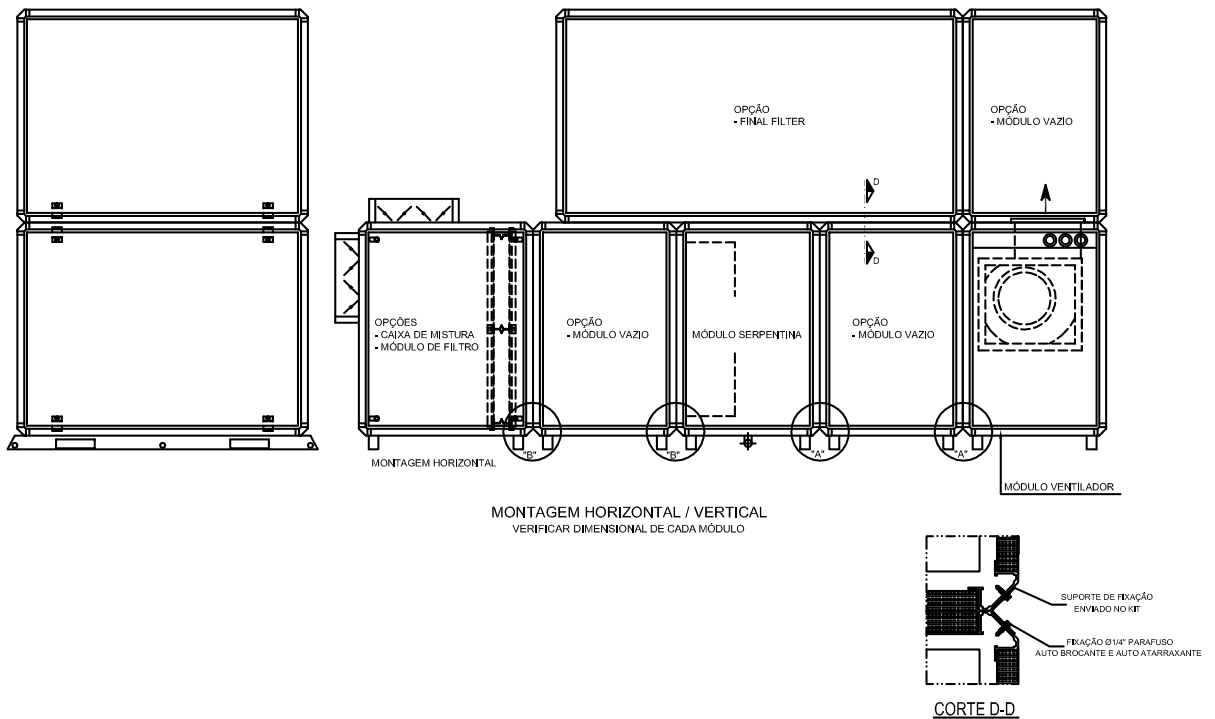
Fig. XVIII - 18 - Montagem Horizontal com Final Filter
