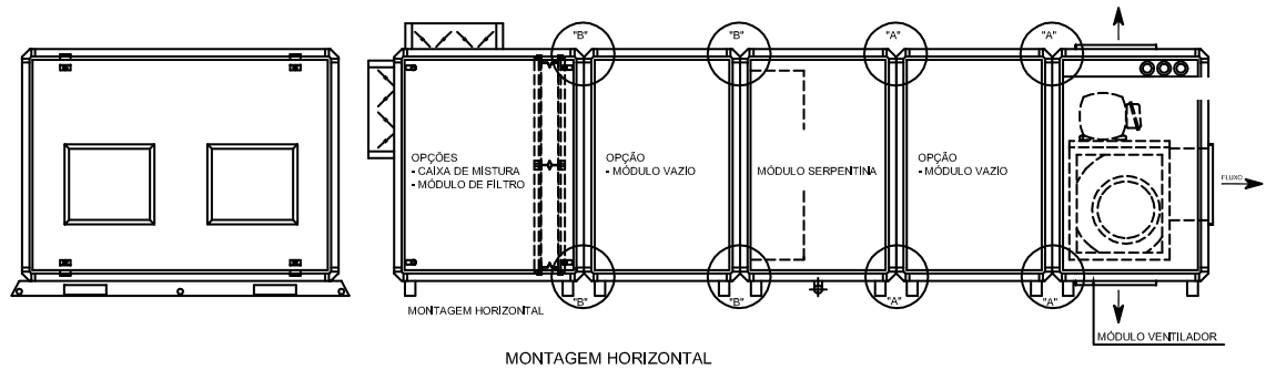
Fig. XVIII - 16 - Montagem Horizontal 05 a 50 - DX/DL
