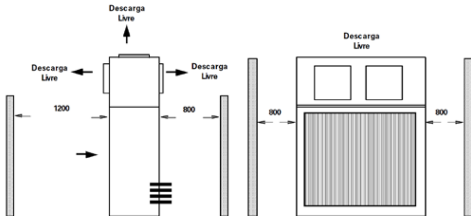
Fig. XVIII 40 - Espaços sugeridos para manutenção e circulação de ar. Unidade condensadora TRCE 050 a 150.
