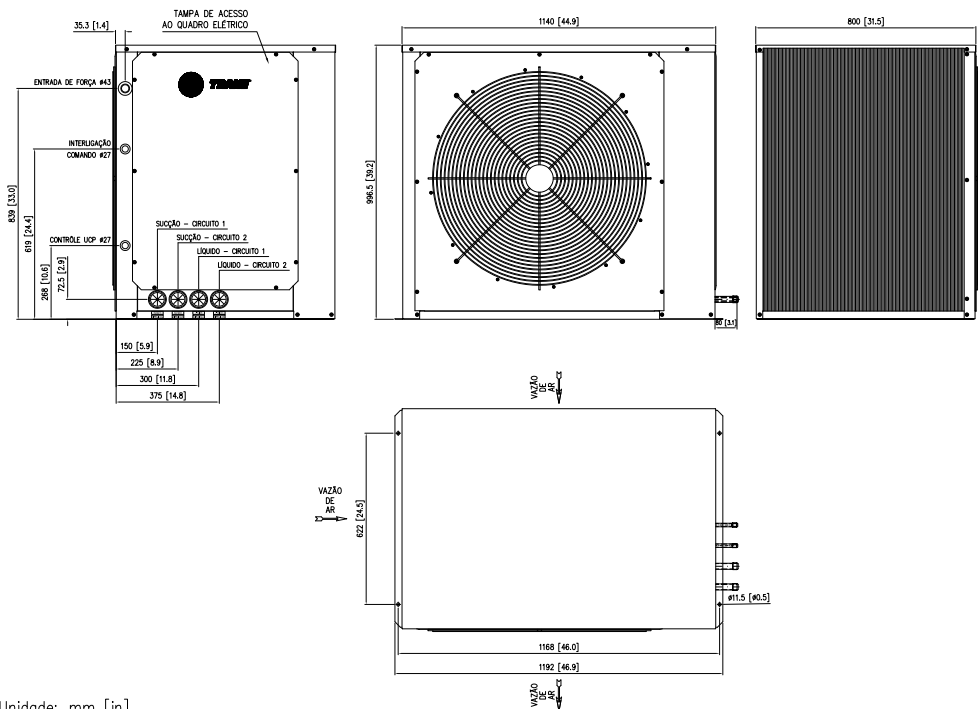
Fig. XVIII-30 - Dimensional Unidades Condensadoras TRAE 100 - 2 circuitos
