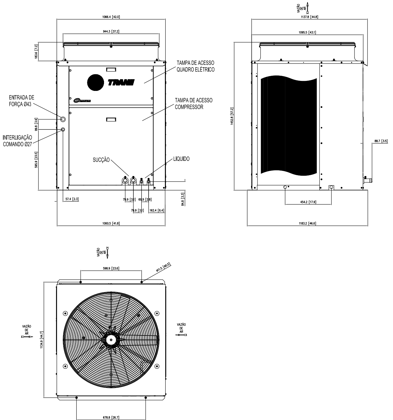
Fig. XVIII-34 - Dimensional Unidades Condensadoras TRAE 200 - 2 circuitos
