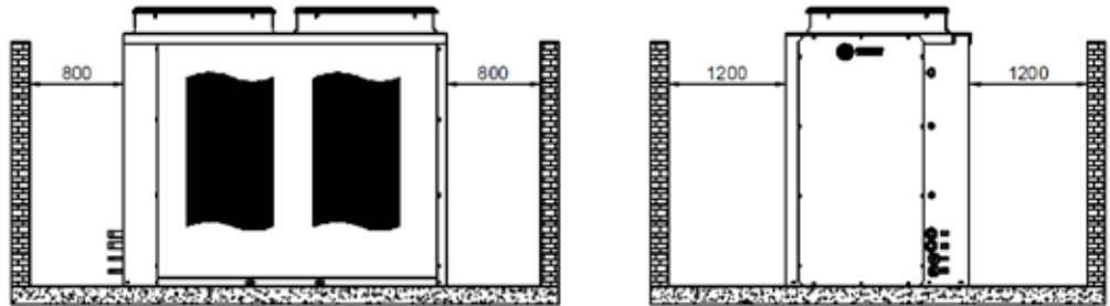
Fig. XVIII 40 - Espaços sugeridos para manutenção e circulação de ar. Unidade condensadora TRCE 050 a 150.
