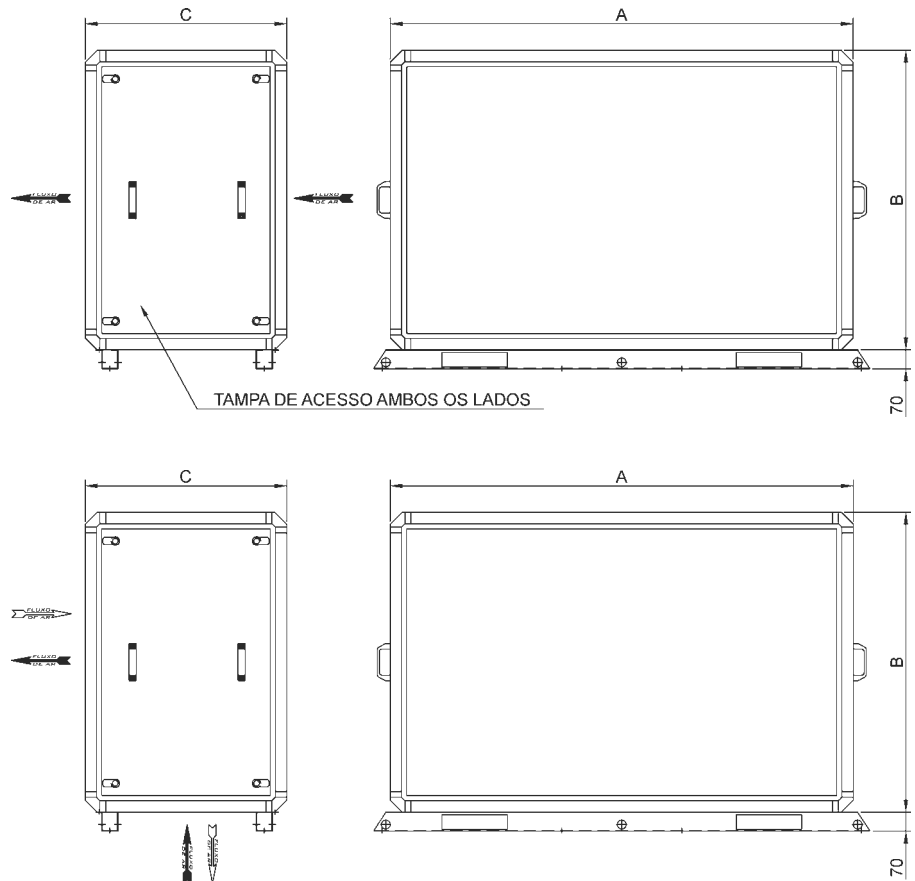
Fig. XVIII 01 - Cotas Módulo Vazio 05 a 50 (DX e DL)
