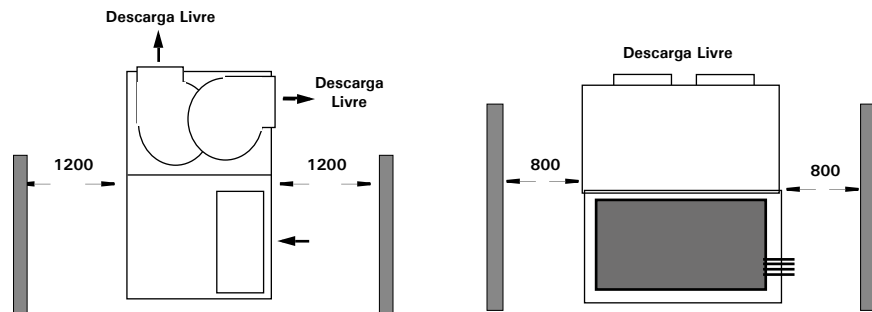
Fig. XVIII-25 - Espaços sugeridos para manutenção e circulação de ar para os módulos serpentina e ventilador. (Gabinete Vertical)
