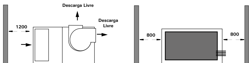
Fig. XVIII-26 - Espaços sugeridos para manutenção e circulação de ar para os módulos serpentina e ventilador. (Gabinete Horizontal)
