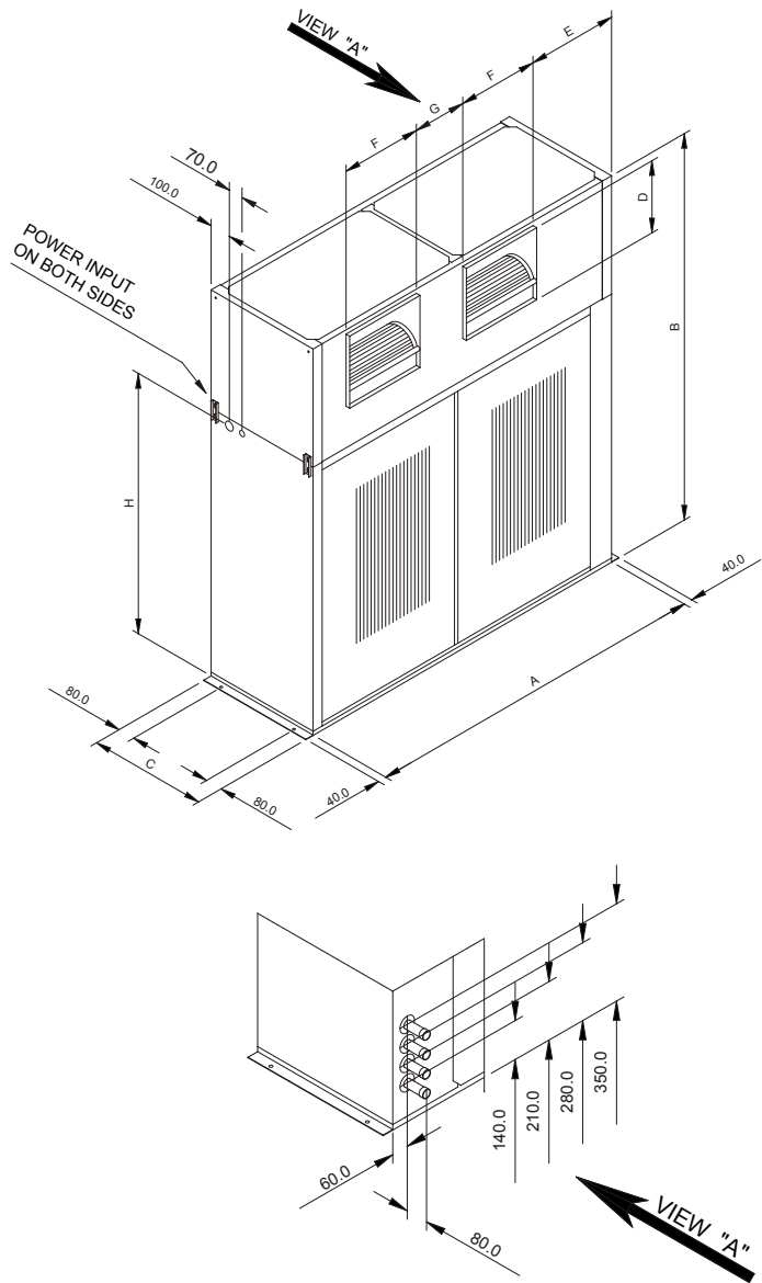
Fig. X 35 - Dimensions TRCE
