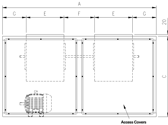
Fig. 17 - Dimensional Data - Fan Module - 200 to 300
