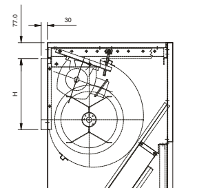
OPÇÃO DESCARGA HORIZONTAL TRASEIRA CAPAC. 100/125/150
