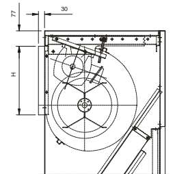
OPÇÃO DESCARGA HORIZONTAL TRASEIRA CAPAC. 100/125/150
