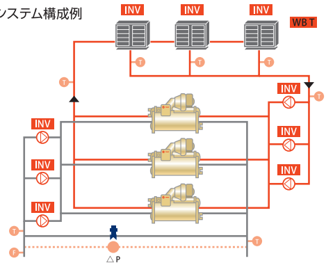
システム構成例
