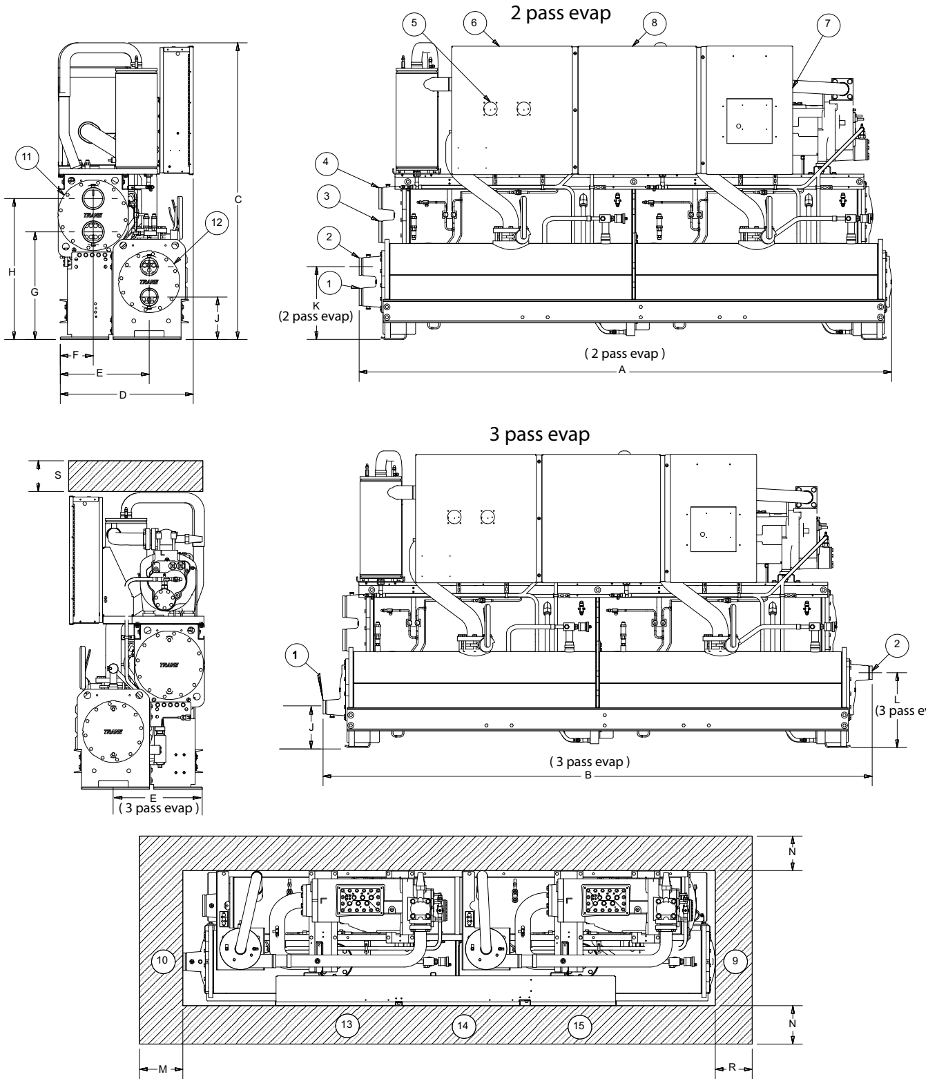
Figure 6. RTWD - 50 Hz dimensions - 70-150 ton SE, 60-120 ton HE
